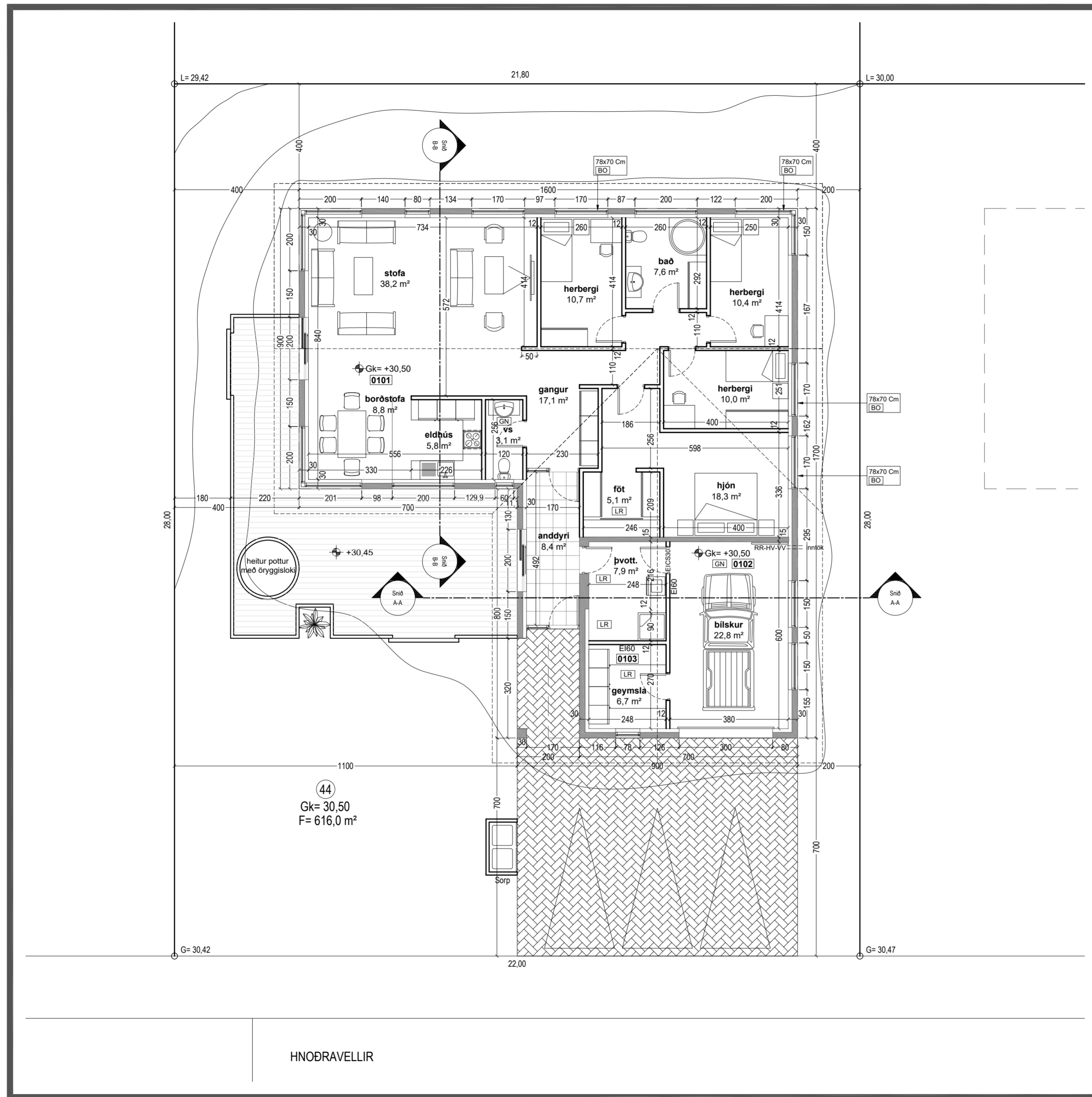
Grunnmynd 1:100
